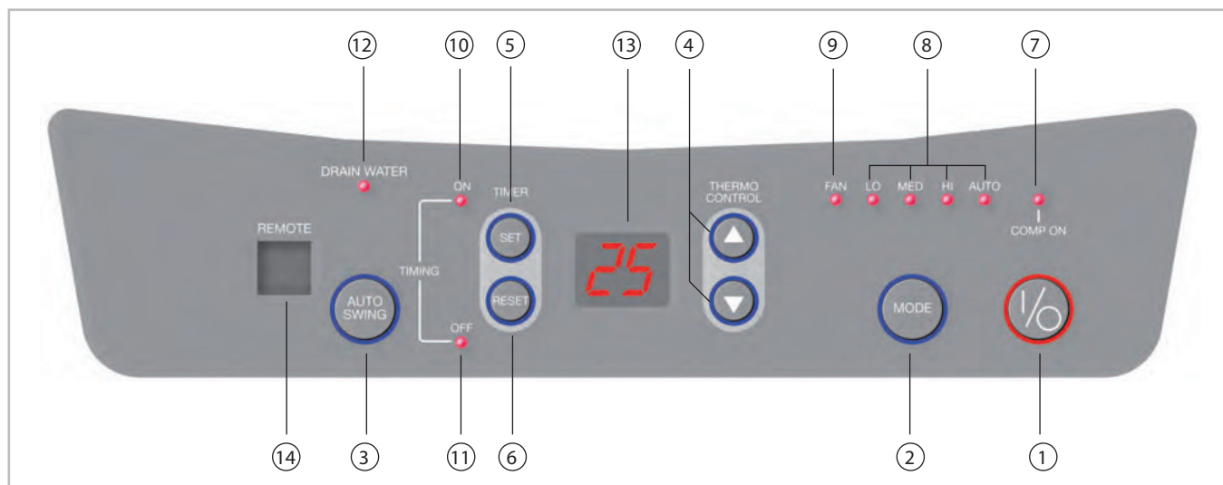
Obr. 3: Ovládací panel
