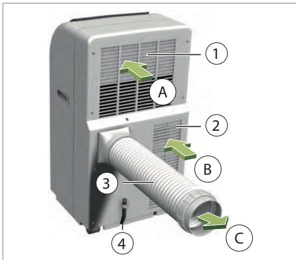
Obr. 2: Pohled zezadu
